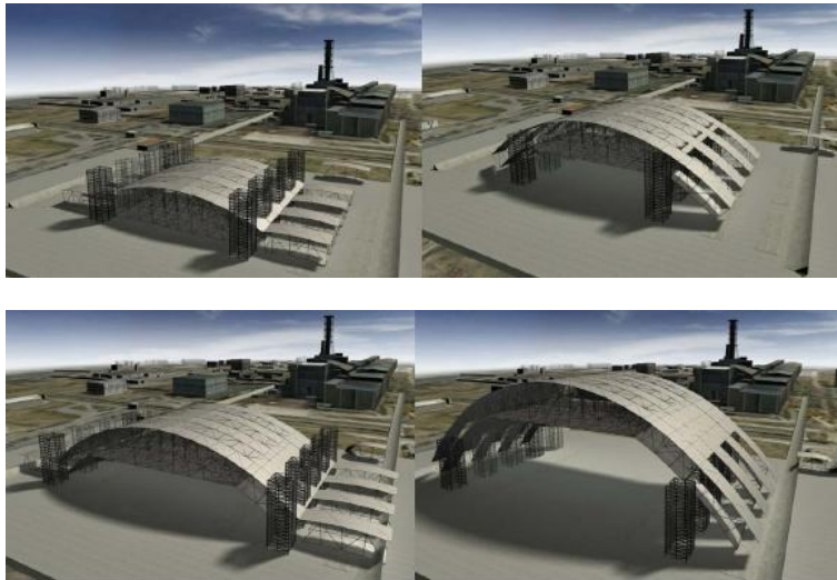
Схема монтажных операций (проект)
