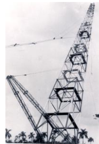
Куба, монтаж опрокидыванием
